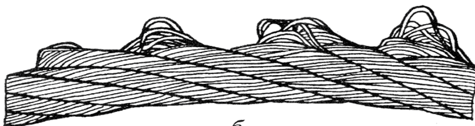
Рисунок 5. Выдавливание проволок прядей: а - в одной пряди; б - в нескольких прядях
