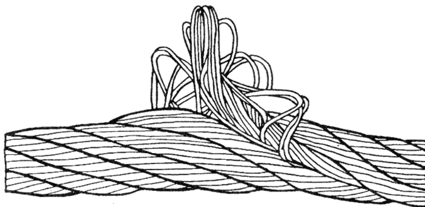
Рисунок 4. Выдавливание сердечника
